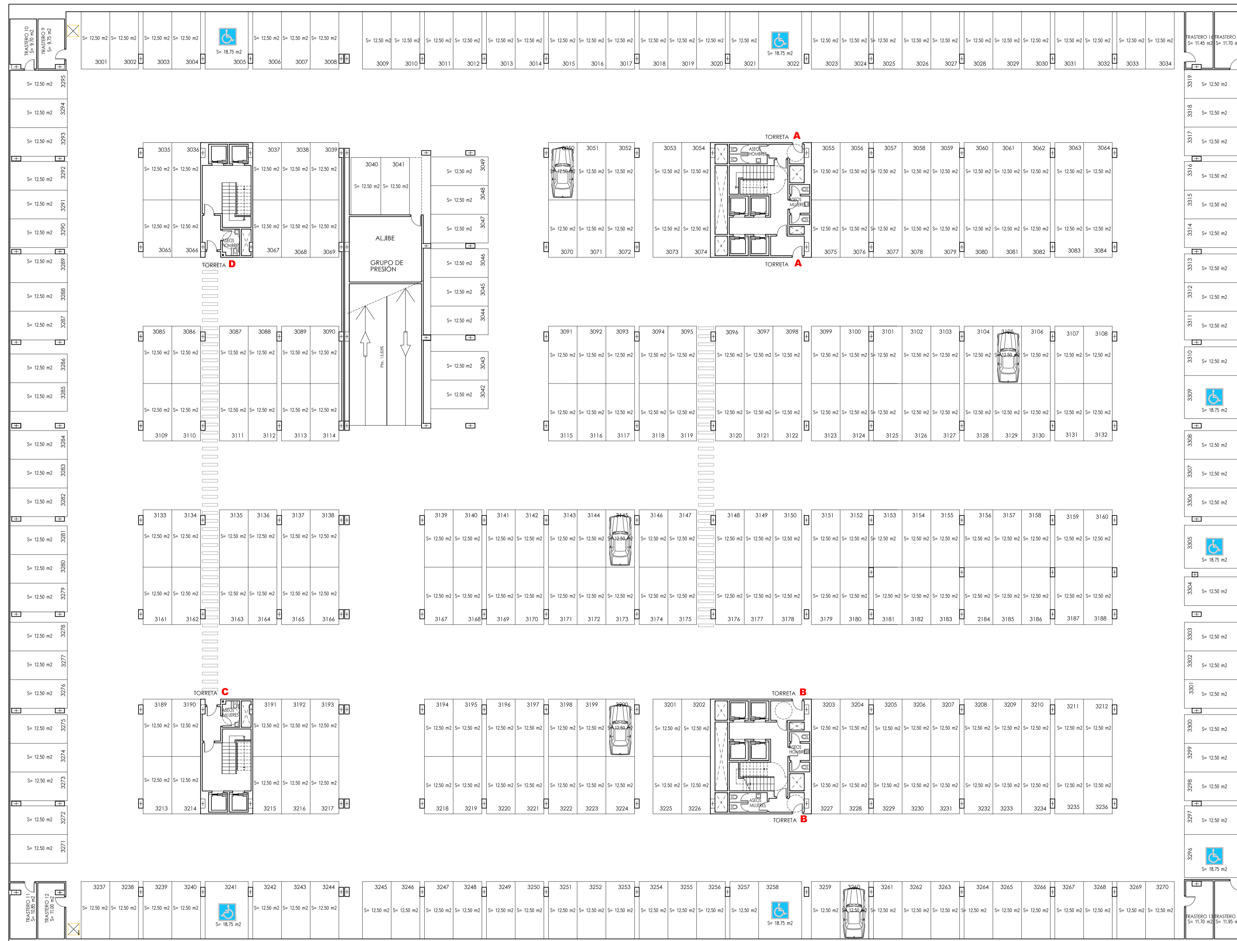
PLANTA SOTANO -3
